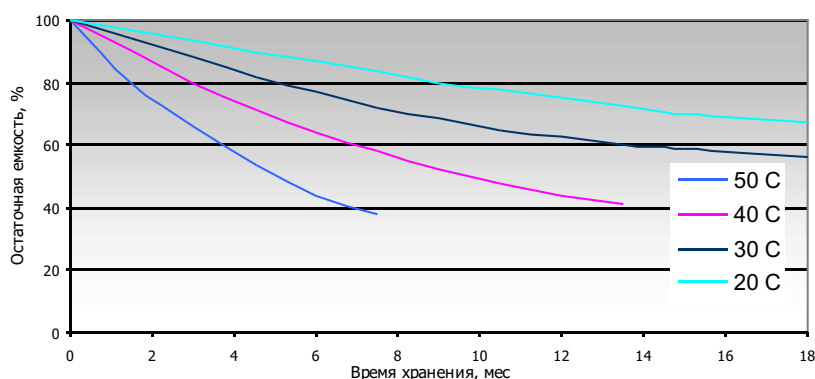
Характеристики саморазряда
